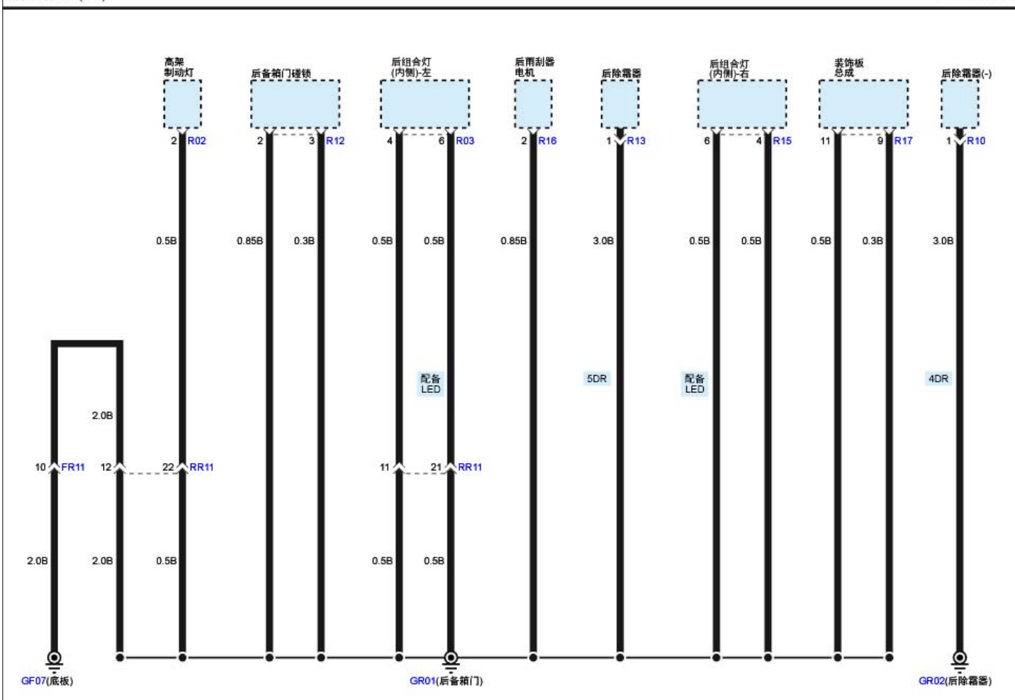
搭铁分布(12)
